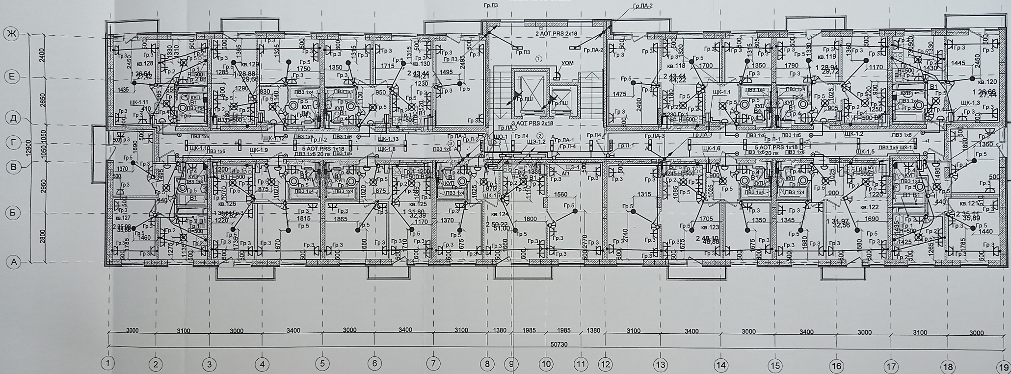
План 10-го этажа
